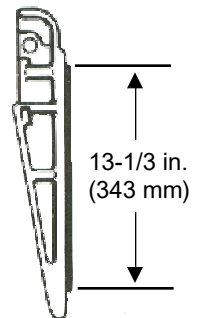
CMS-XL Grip Length
